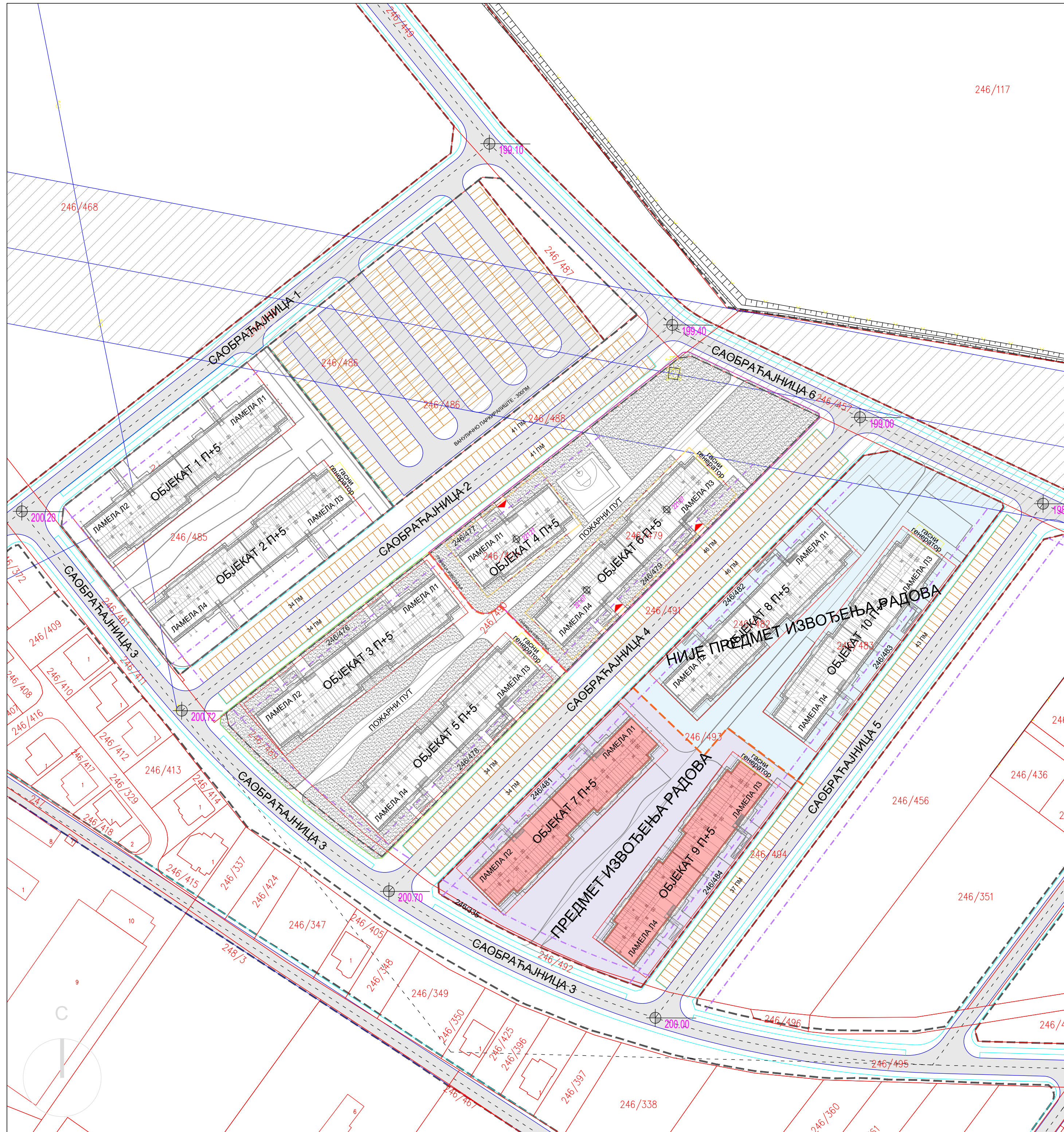
ПЛАН ОБУХВАТА ИЗВОЂЕЊА РАДОВА УНУТАР БЛОКОВСКОГ УРЕЂЕЊА НА ДЕЛУ КП.246/493 ВЕЗАНО ЗА ОБЈЕКТЕ 7 И 9.
