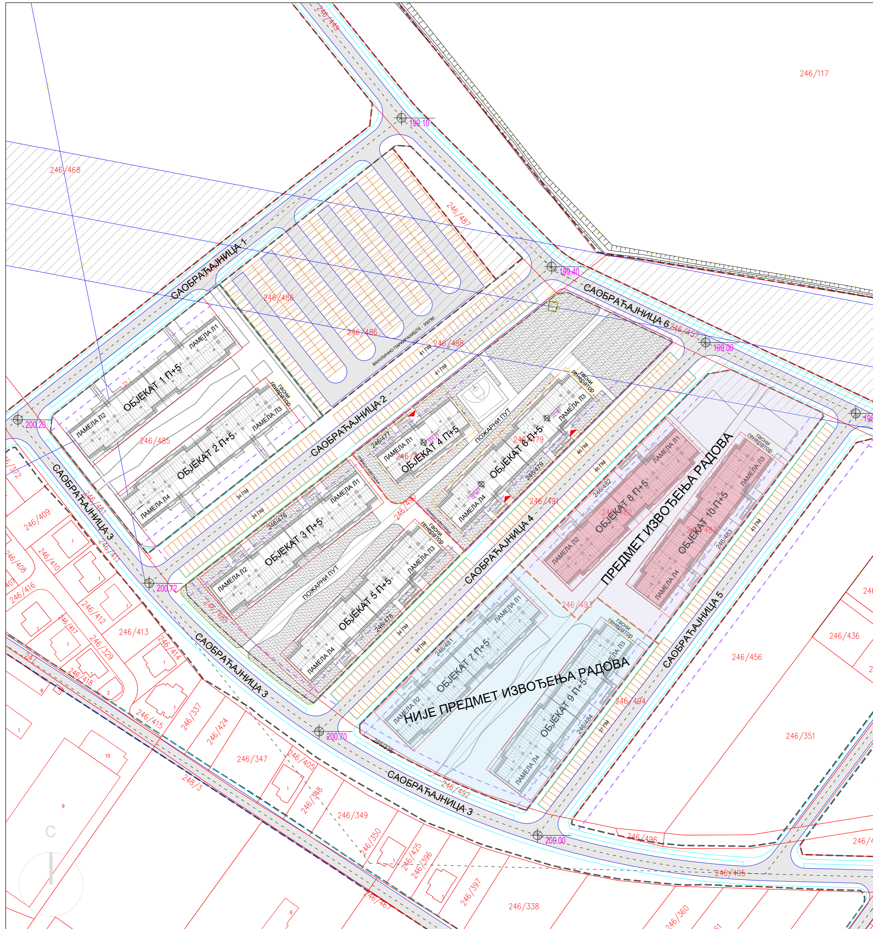
ПЛАН ОБУХВАТА ИЗВОЂЕЊА РАДОВА УНУТАР БЛОКОВСКОГ УРЕЂЕЊА НА ДЕЛУ КП.246/493 ВЕЗАНО ЗА ОБЈЕКТЕ 8 И 10.
