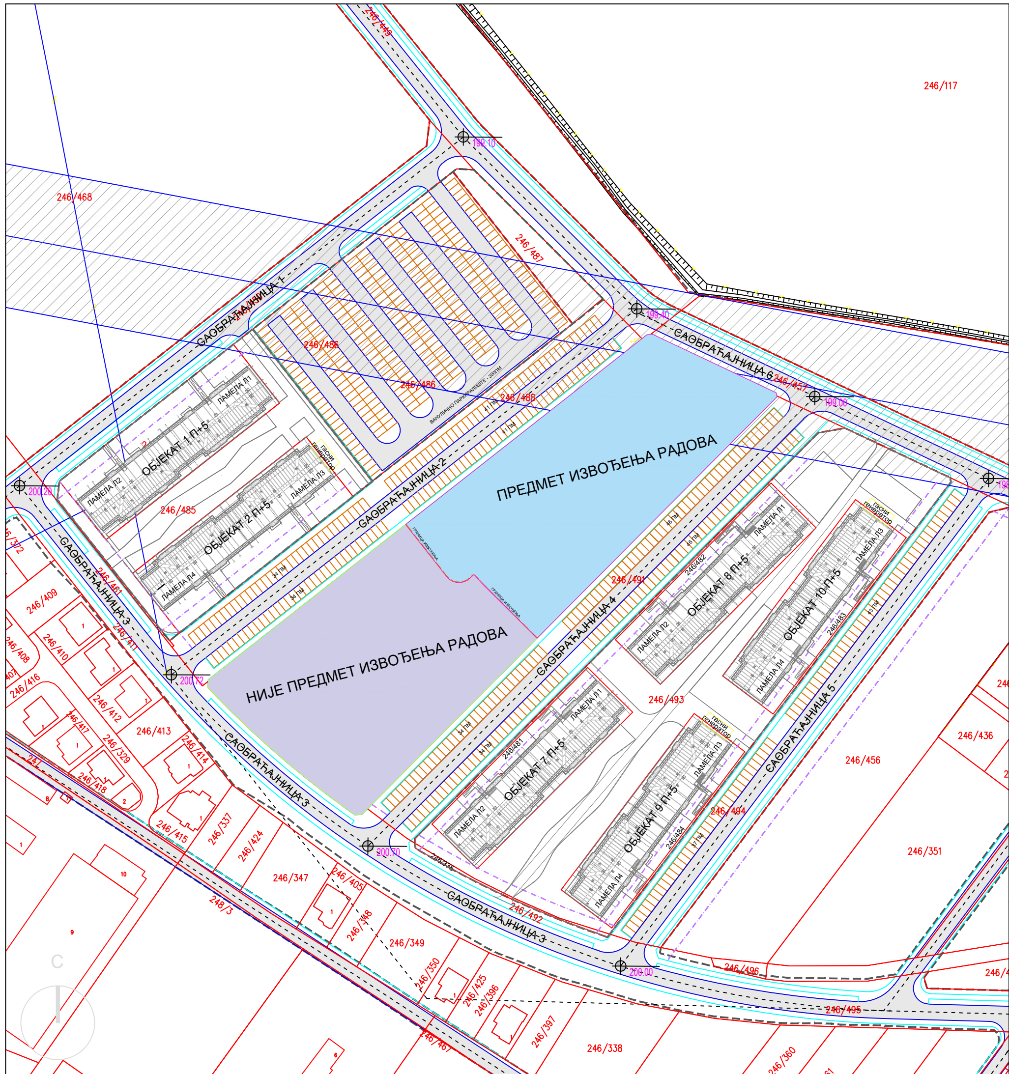
ПЛАН ОБУХВАТА ИЗВОЂЕЊА РАДОВА УНУТАР БЛОКОВСКОГ УРЕЂЕЊА НА ДЕЛУ КП.246/490
